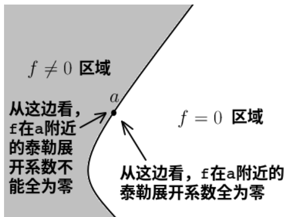
Figure 4.2: 解析函数不能存在整片的恒为零区域和非零区域连通并存的情况, 否则公共边界上无法进行泰勒展开
